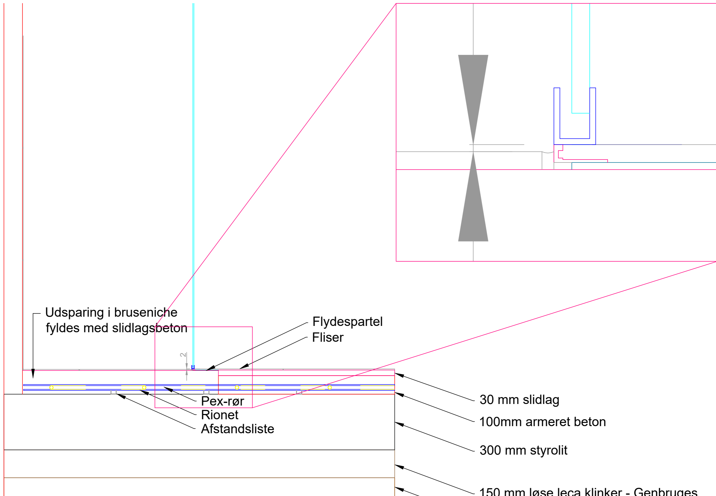
Detalje B - Gulvopbygning
