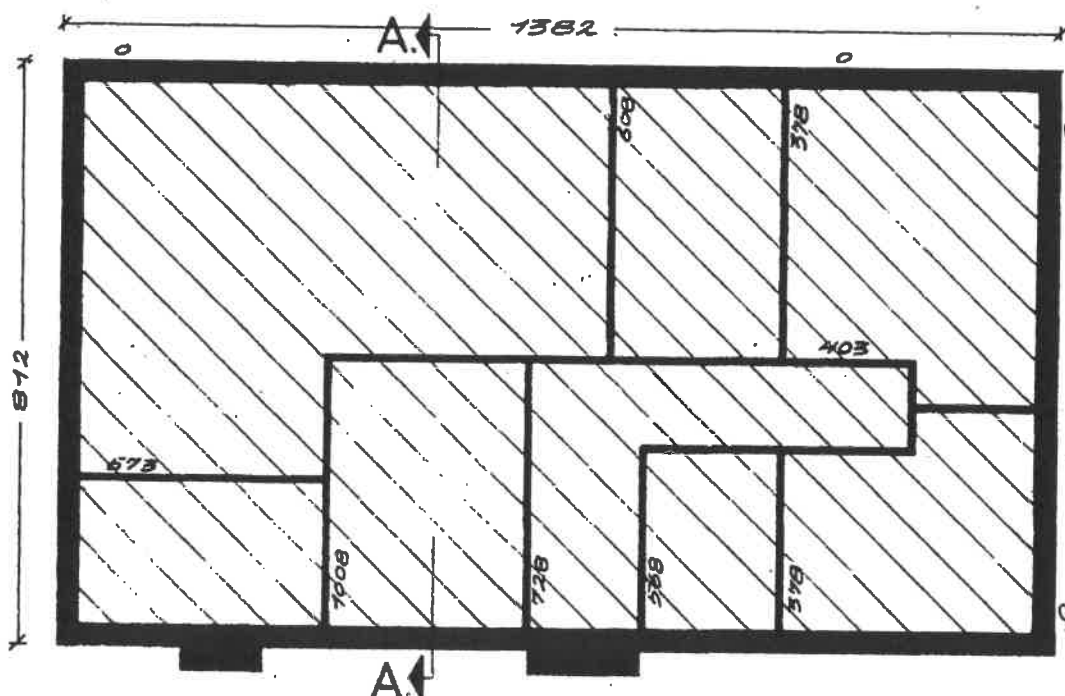
SOKKELPLAN
