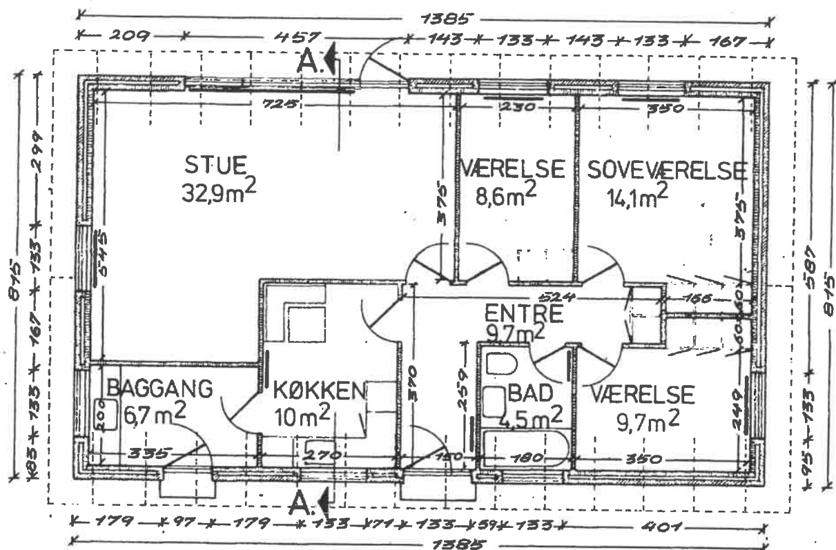
STUEPLAN
