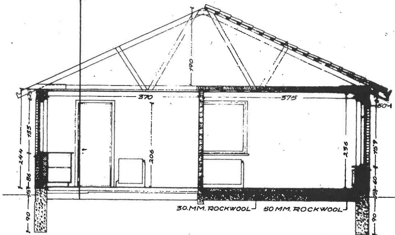
SNIT. A-A.
