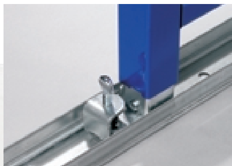
Fastgørelse i Duofix System gulvskinne
