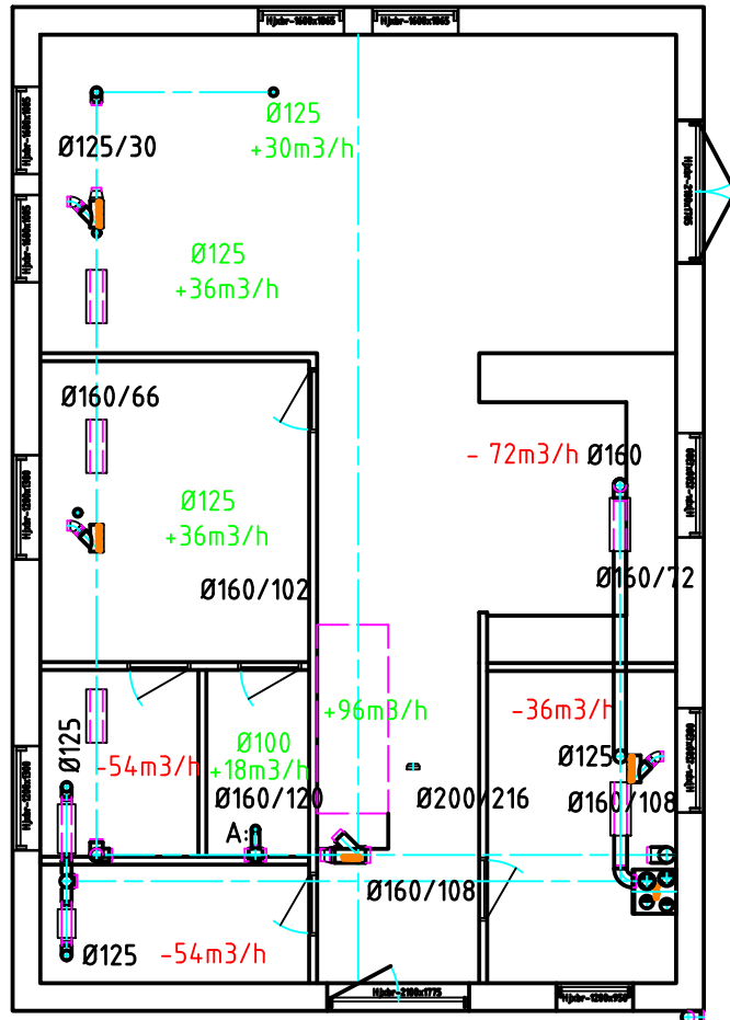
Stueplan
