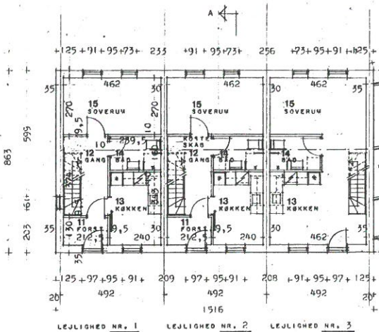
LEJLIGHED NR. 1 LEJLIGHED NR. 2 LEJLIGHED NR. 3
