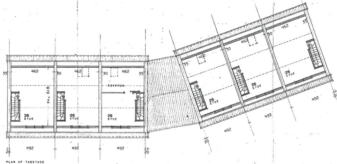
PLAN AF TAGETAGE
