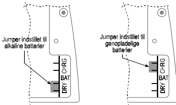
Figure 14. Indstilling af batteritypewælger
