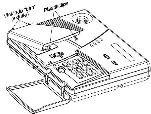
Figur 11. Fjern dækslet
