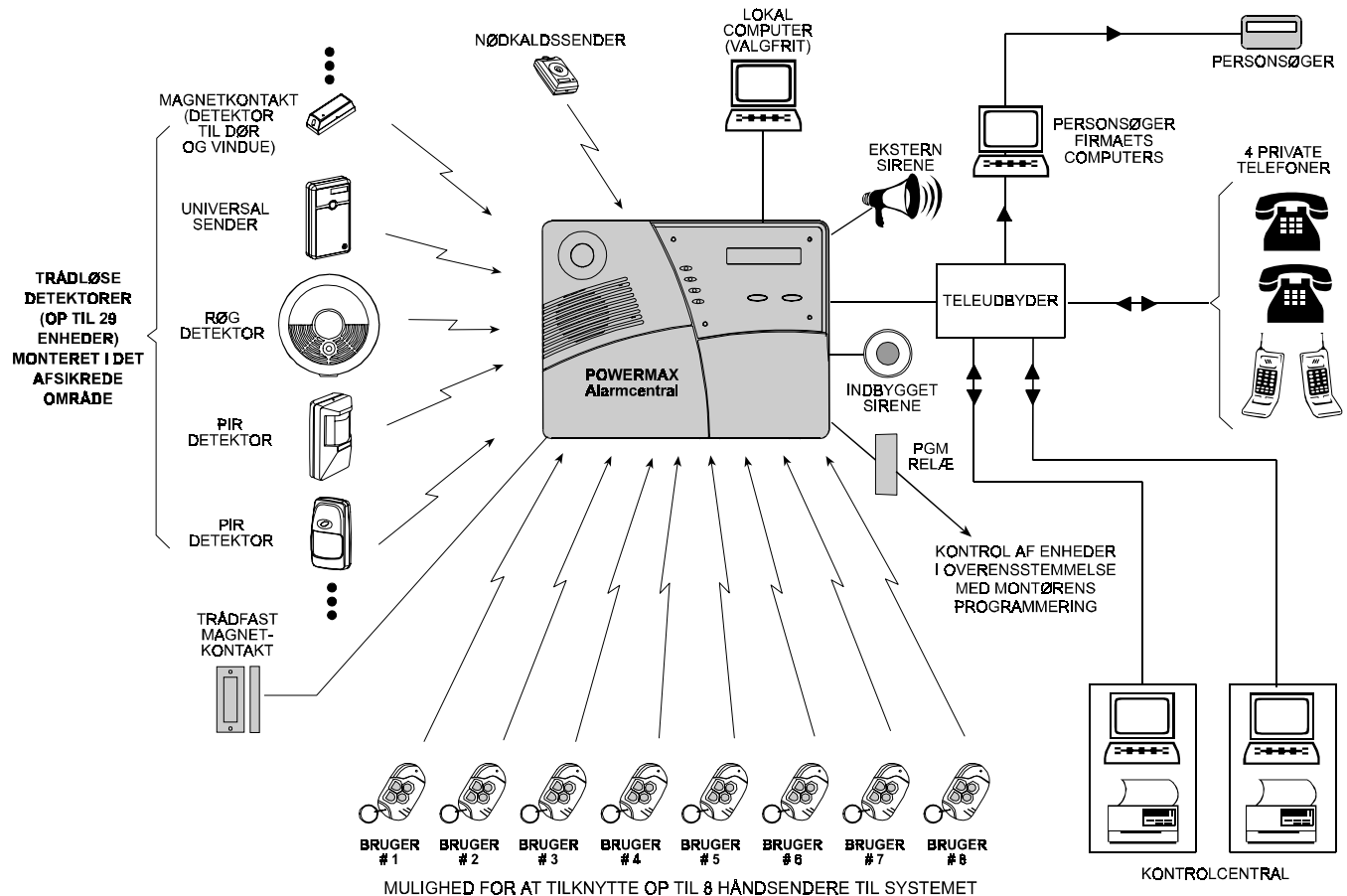
Figur 2. Typisk systemopsætning
