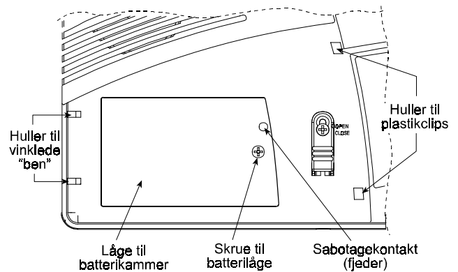
Figur 12. Batterikammer låge
