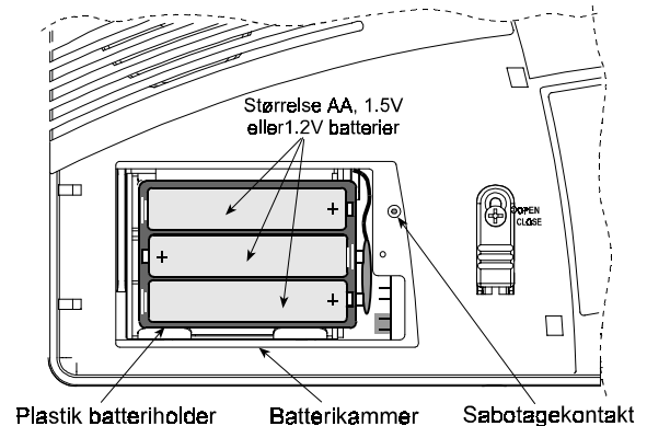
Figur 13. Batterikammer og batteriholder
