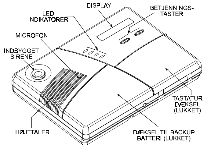
Figur 1. Alarmcentral med dækslerne lukket
