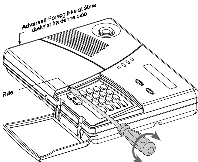
Figur 10. Åbne dækslet
