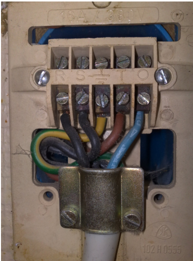
Min 16A 380v ledning i væg =R, S, T, O og jordledning
