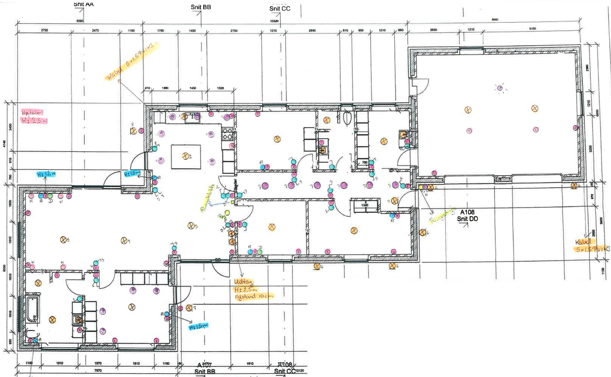
1 B. Grundplan 1-75 1:75
